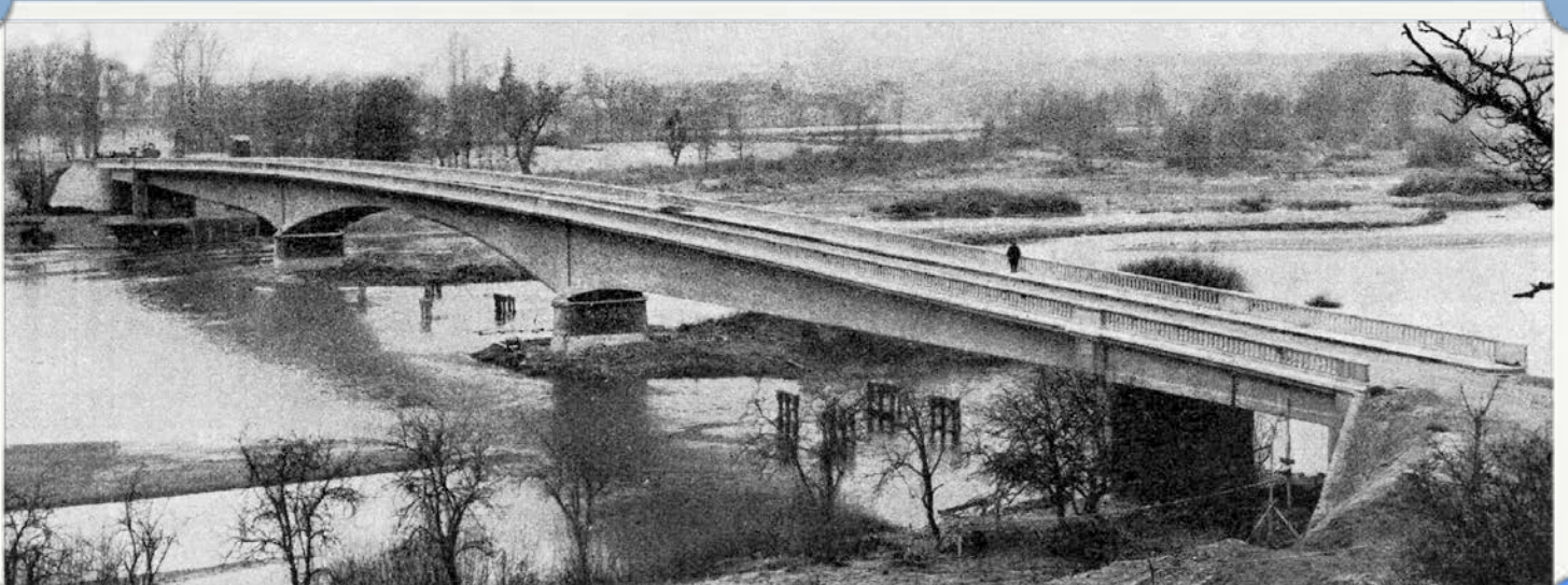
1948 - Pont cantilever
